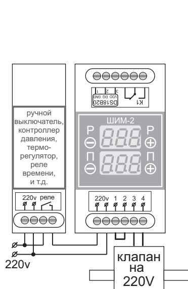
Рис. 1. Вариант подключения прибора в режиме P1. Старт-стопы для клапана отбора формирует внешнее устройство.
