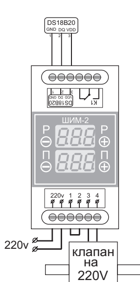
Рис. 2. Вариант подключения прибора в режиме P2. Старт-стопы для отбора формирует встроенный термоконтроллер t_1 .
