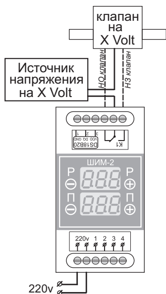
Рис. 4. Вариант подключения к прибору клапана с катушкой не на 220V, а также НО-клапана, в режимах P1 и P2 и P3 с Рт.
