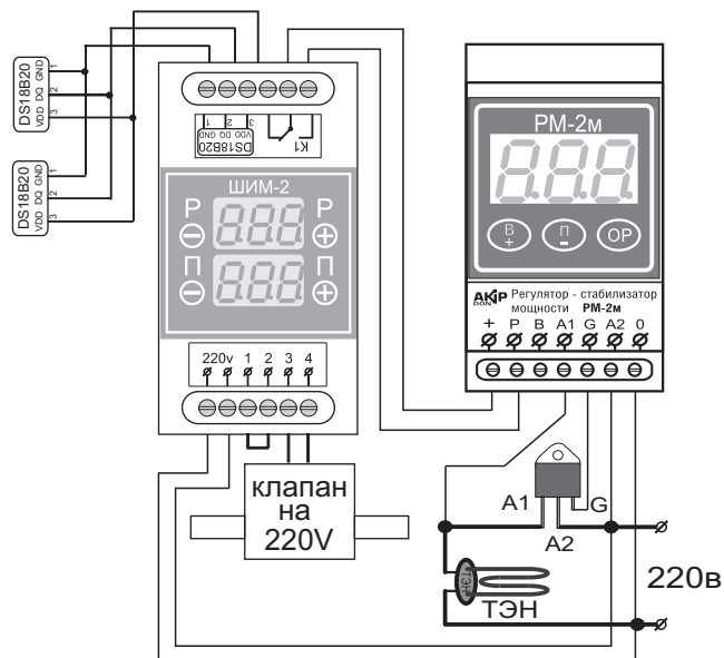
Рис. 3. Вариант подключения прибора в режиме P3. Терморегулятор t_2 прибора ШИМ-2 используется для управления режимом разгона РМ-2м.
